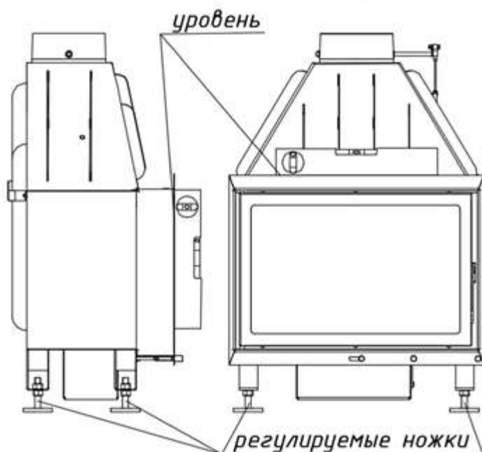
Схема установки топки по уровню
